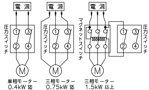
結線図一例 (接点構成2bの時)
